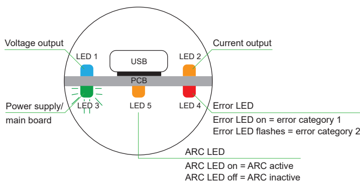
Fig. 40 Status LEDs
