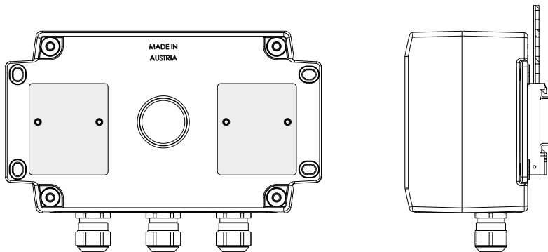
Fig. 26 DIN rail installation
